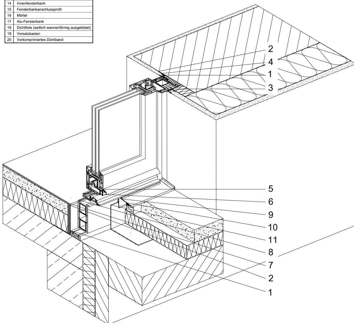
Bild 5.6: Darstellung der Abdichtung Anschluss barrierefreie Fenstertür/Laibung außen
