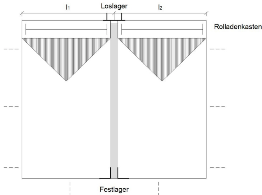
Bild 3.4: Darstellung von geteilten Fensterkonstruktionen mit Rollladenanlagen und Anschluss an ein Loslager
