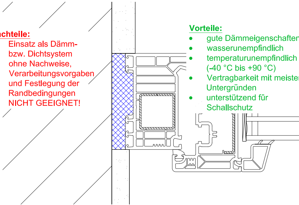
Bild 4.16: Darstellung der Vor- und Nachteile bei Einsatz von Schäumen als Dämm- bzw. Dichtstoff im Fugenbereich
