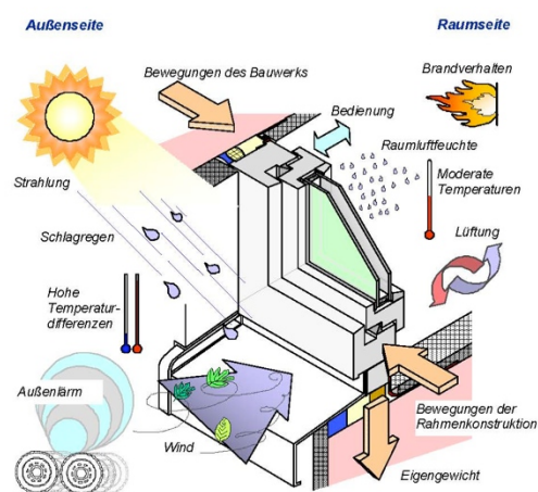
Bild 2.1: Schematische Darstellung der Einwirkungen auf ein Fenster [1]
