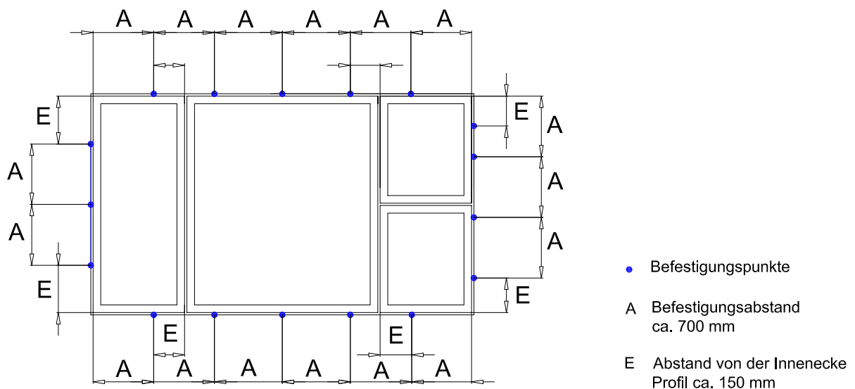
Bild 3.2: Befestigungsabstände
