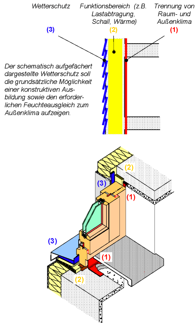
Bild 2.2: Ebenenmodell und Übertragung auf die Anschlussfuge [1]
