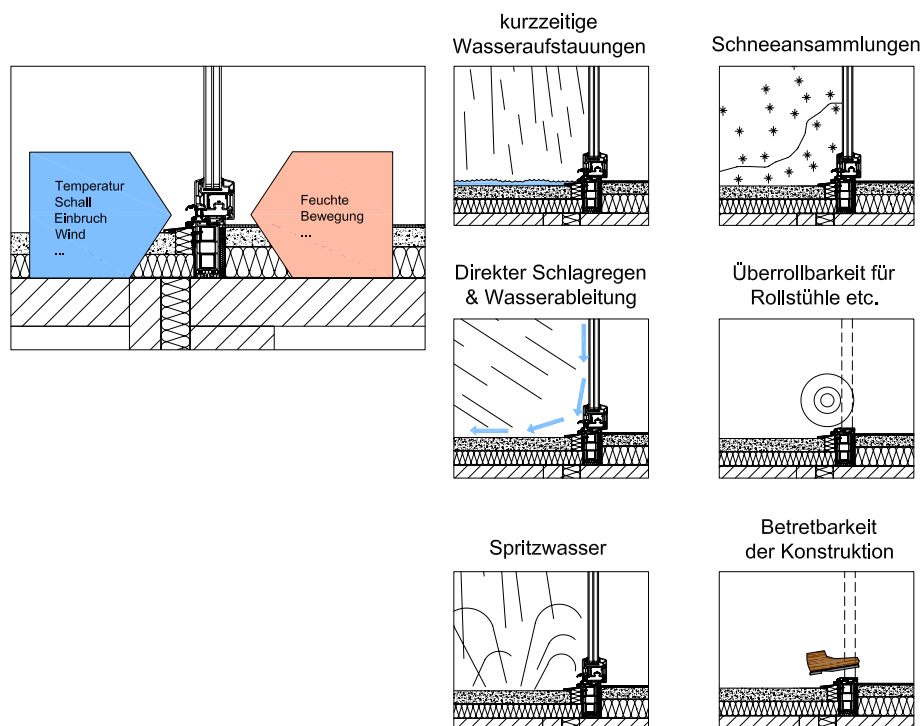
Bild 4.8: Unterschiedliche Belastungen und Anforderungen an den Bodenanschluss bzw. die Schwellenausbildung bei feststehenden und offenen Elementen
