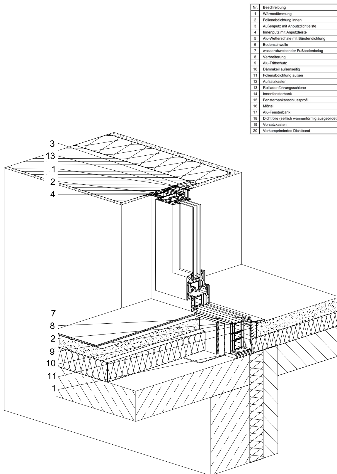
Bild 5.8: Darstellung der Abdichtung bei Anschluss Fenstertür/Laibung innen
