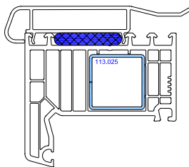
1x Blendrahmen mit Standardaussteifungsprofil ≥ 1x erforderlich
