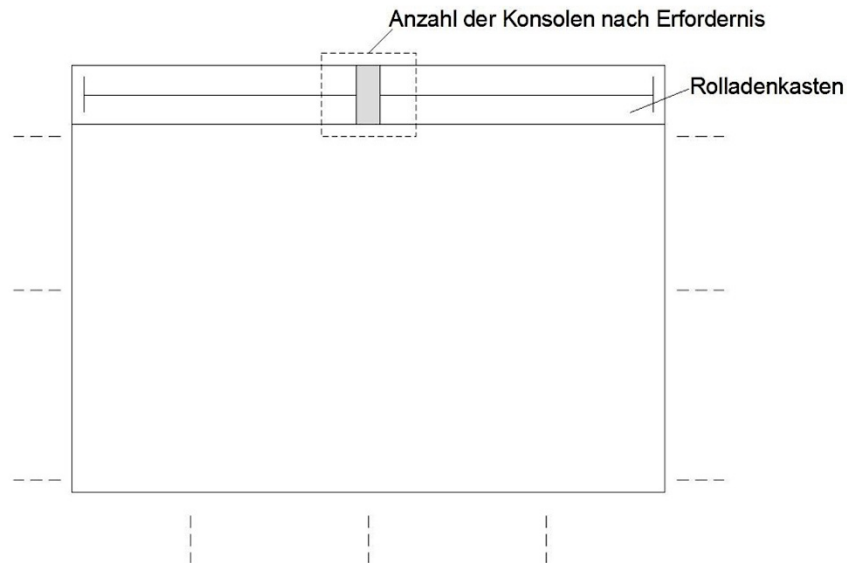
Bild 3.6: Darstellung einer weitgespannten Rollladenanlage mit Einsatz einer tragenden Konsole
