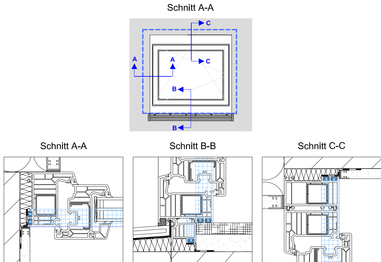
Bild 4.6: Beispiel einer raumseitigen luftdichten Abdichtung eines Kunststofffensters mit Profillinie im Anschlussbereich Laibung, Brüstung und Sturz mit Verbreiterung
