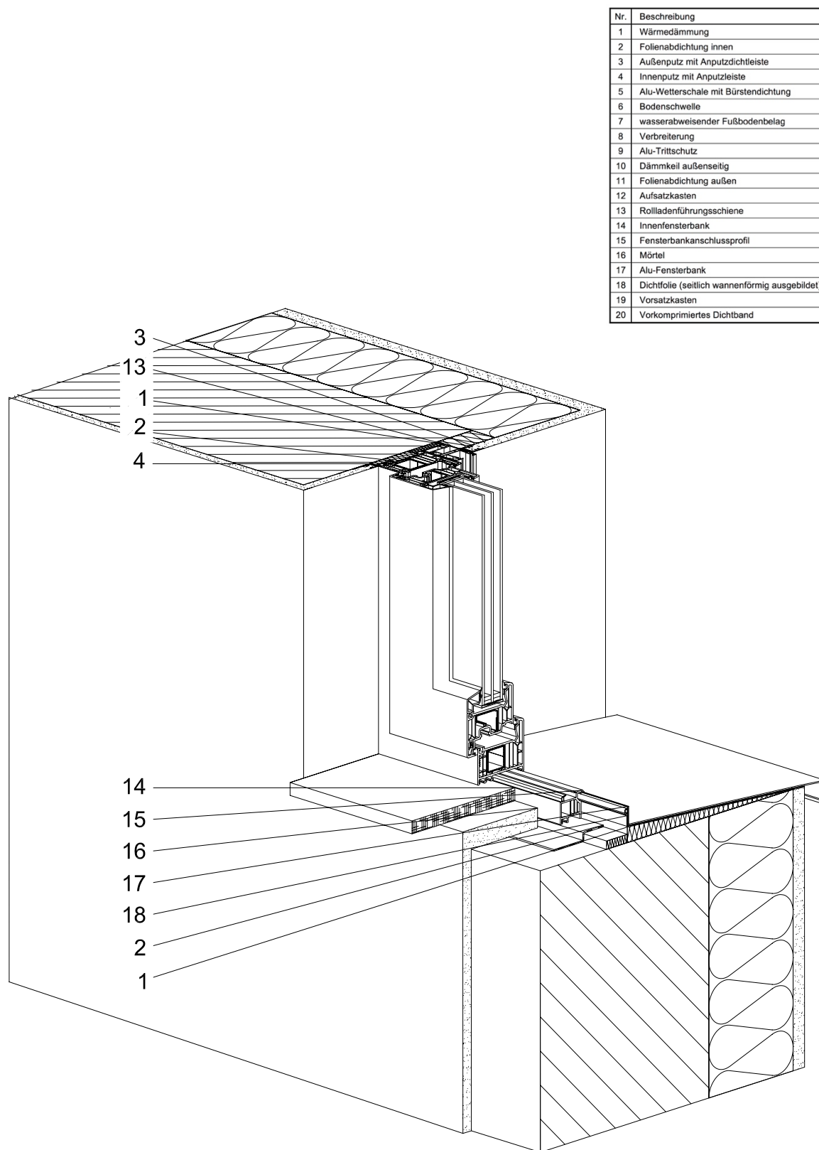
Bild 5.12: Darstellung der Abdichtung bei Anschluss Brüstung/Laibung innen
