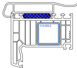
1x Blendrahmen mit Sonderaussteifungsprofil ≥ 1x erforderlich
