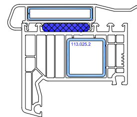
1x Blendrahmen mit Sonderaussteifungsprofil + 1x Zusatzaussteifung ≥ 1x erforderlich
